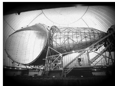
L'antenne - cornet sous le radôme
